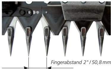
Mittelschnittbalken
