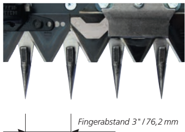
Normalschnittbalken
