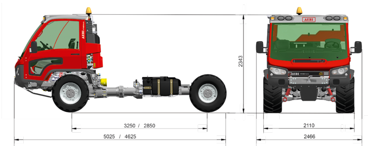
Aebi VT450 Vario
