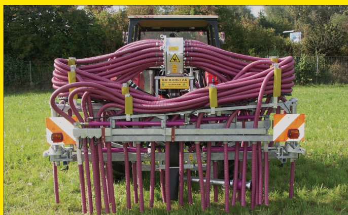
Transportstellung mit einer Aussenbreite von 275cm
