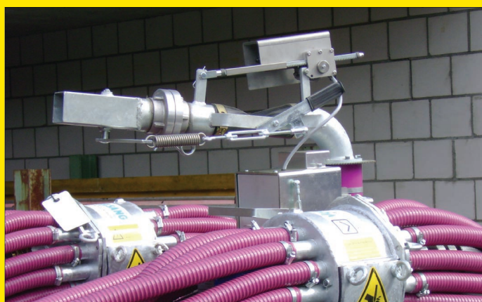
Aufgebaute Weitwurfdüse (Option)
